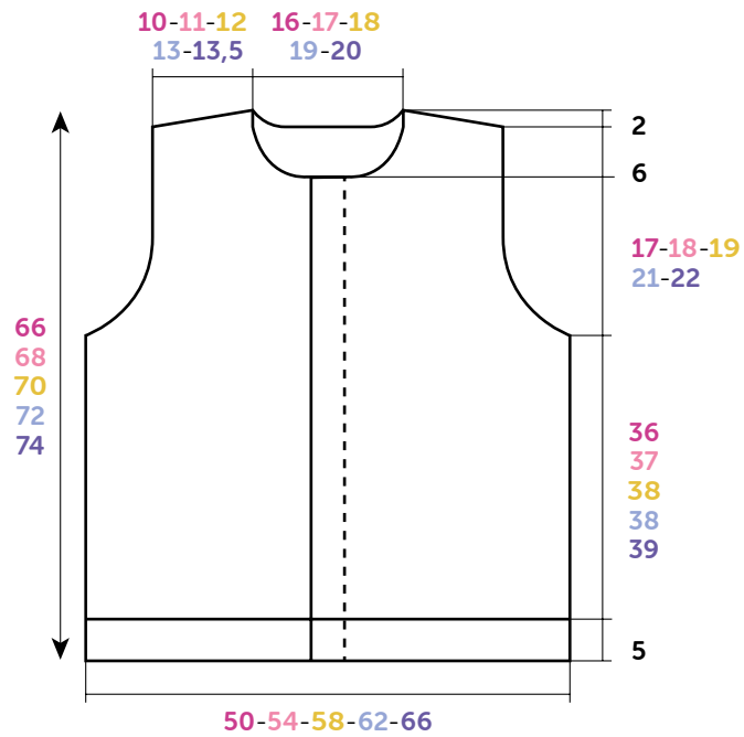
RUGPAND - VOORPANDEN
